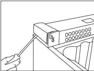
4. Täcklisterna på sockelsidorna demonteras försiktigt med hjälp av en flatslipad skruvmejsel
